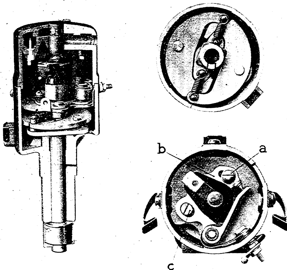
Fig. A. — VUE EN COUPE DE L'ALLUMEUR
