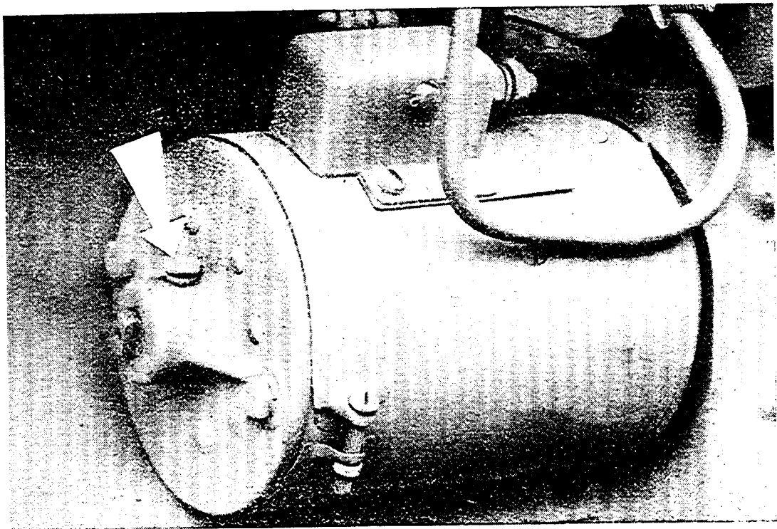
Fig. B. — VUE DU DÉMARREUR (La flèche indique le graisseur du palier AV.)
