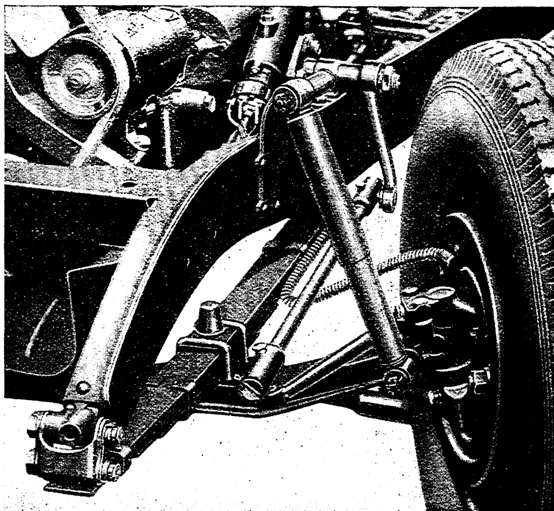
Fig. B. — VUE DE L'ESSIEU AVANT ET DE LA SUSPENSION
