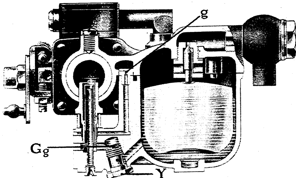
Fig. B. — COUPE DU CARBURATEUR
